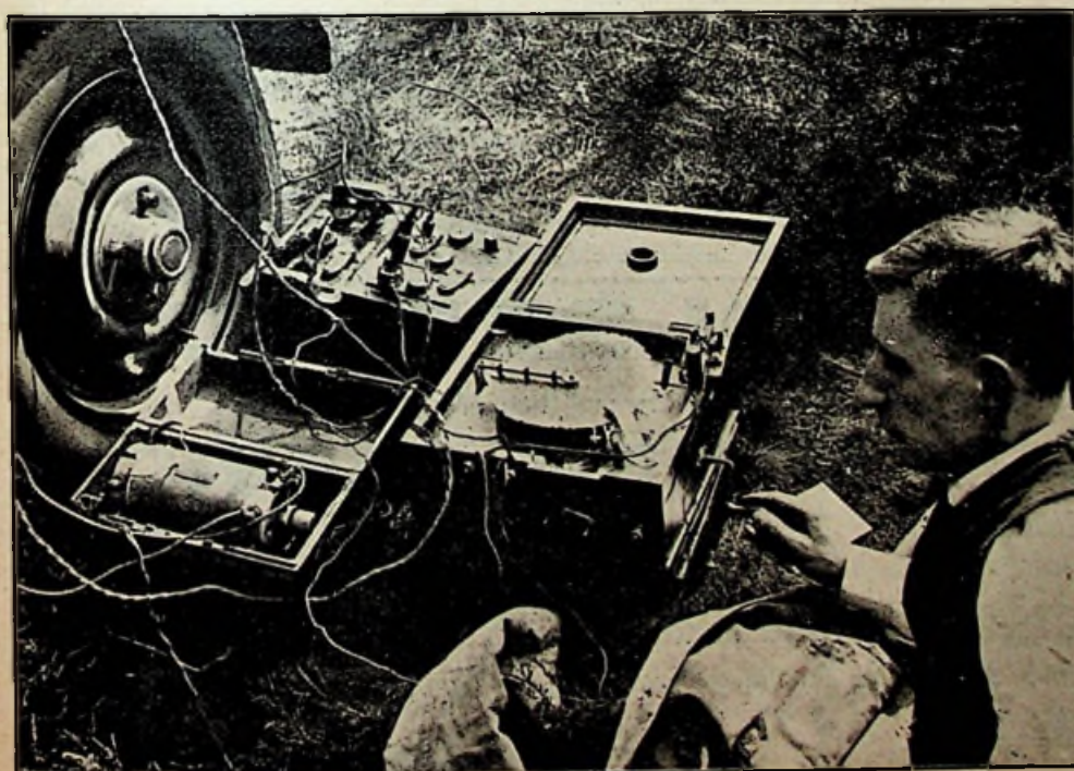
O. M. Otten draait z'n automatische seingever op, daarachter de 1000 V. omvormer.
