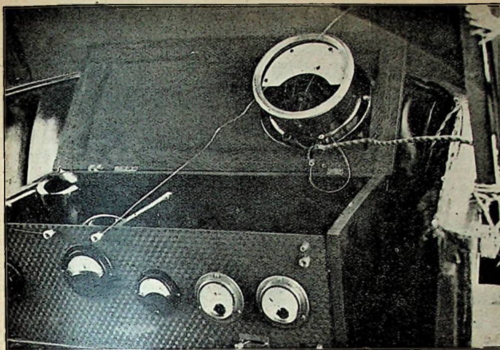
De vos. Links de zendpit MC 1/50. Rechts boven de h.sp.voltmeter
